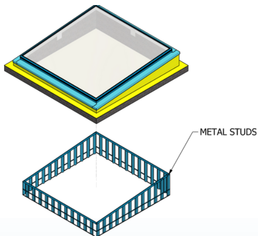
FIG. 2-2 SCALE 1 : 50
