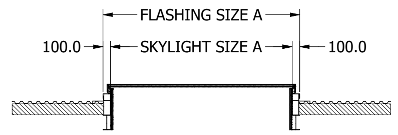
SECTION A-A SCALE 1 : 50
