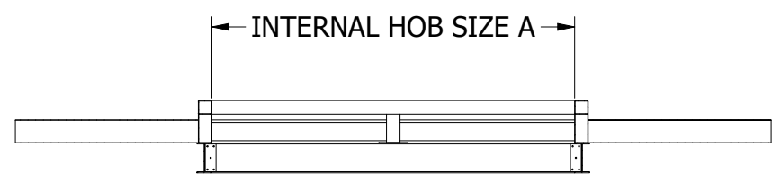
SECTION A-A SCALE 1 : 45
