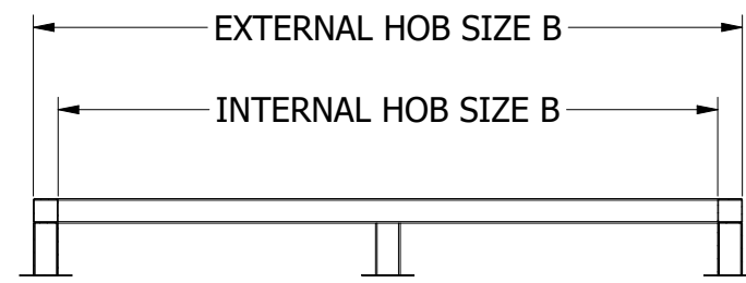
SECTION B-B SCALE 1 : 30
