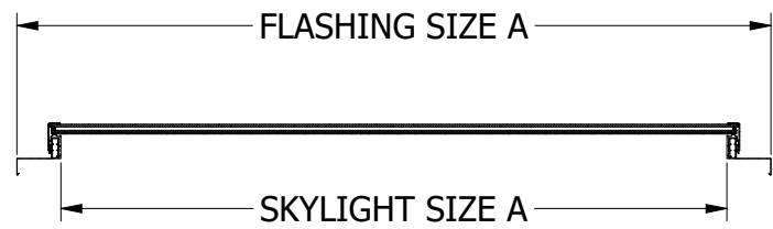
SECTION A-A SCALE 1 : 30
