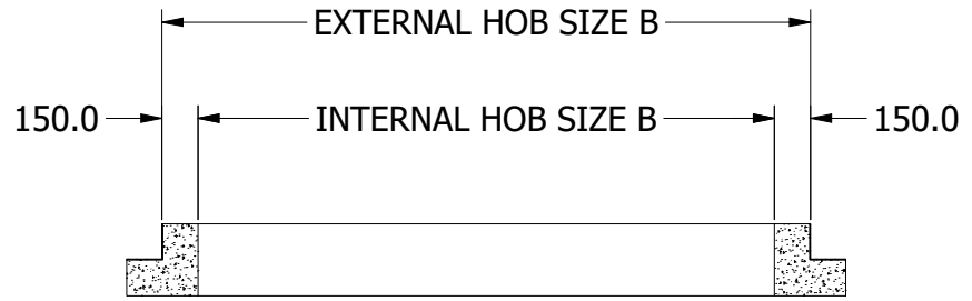
SECTION B-B SCALE 1 : 35
