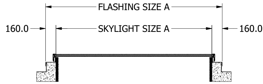
SECTION A-A SCALE 1 : 35
