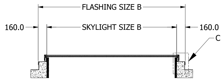
SECTION B-B SCALE 1 : 35
