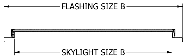
SECTION B-B SCALE 1 : 30
