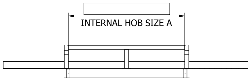
SECTION A-A SCALE 1 : 45
